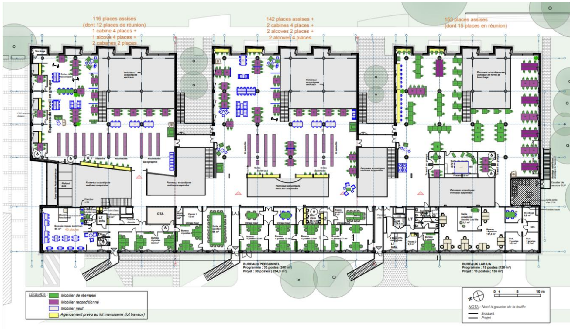
BU Belle-Beille Plan du niveau 1 : salles de travail étudiants et bureaux personnels
