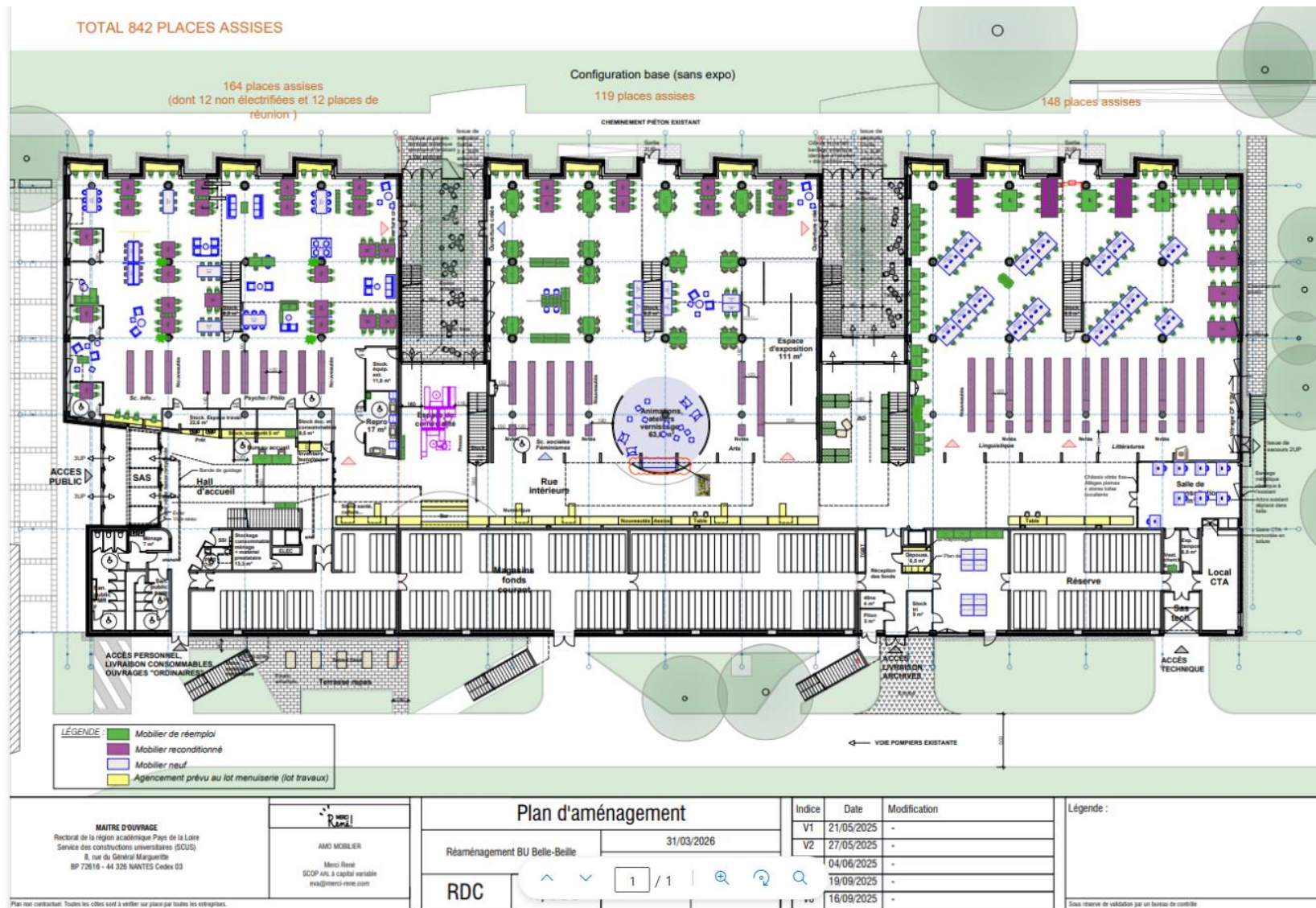
BU Belle-Beille Plan architecte et implantation mobilier rez-de-chaussée, salles de travail, accueil, sanitaires et magasins – jardinets enclos
